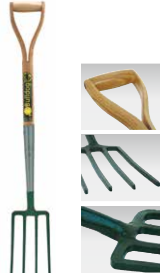
Border Fork 5715042820 ¥18,600 [サイズ] L93.5×W13.2cm [材質] ブレード:カーボンスチール、柄:木(アッシュ)
